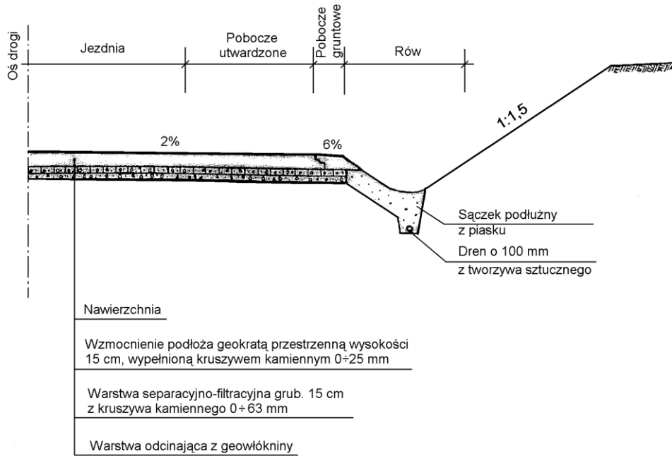
Rys. 4. Przekrój poprzeczny drogi ze wzmocnieniem podłoża geokrąą i kruszywem kamiennym (przykład)
