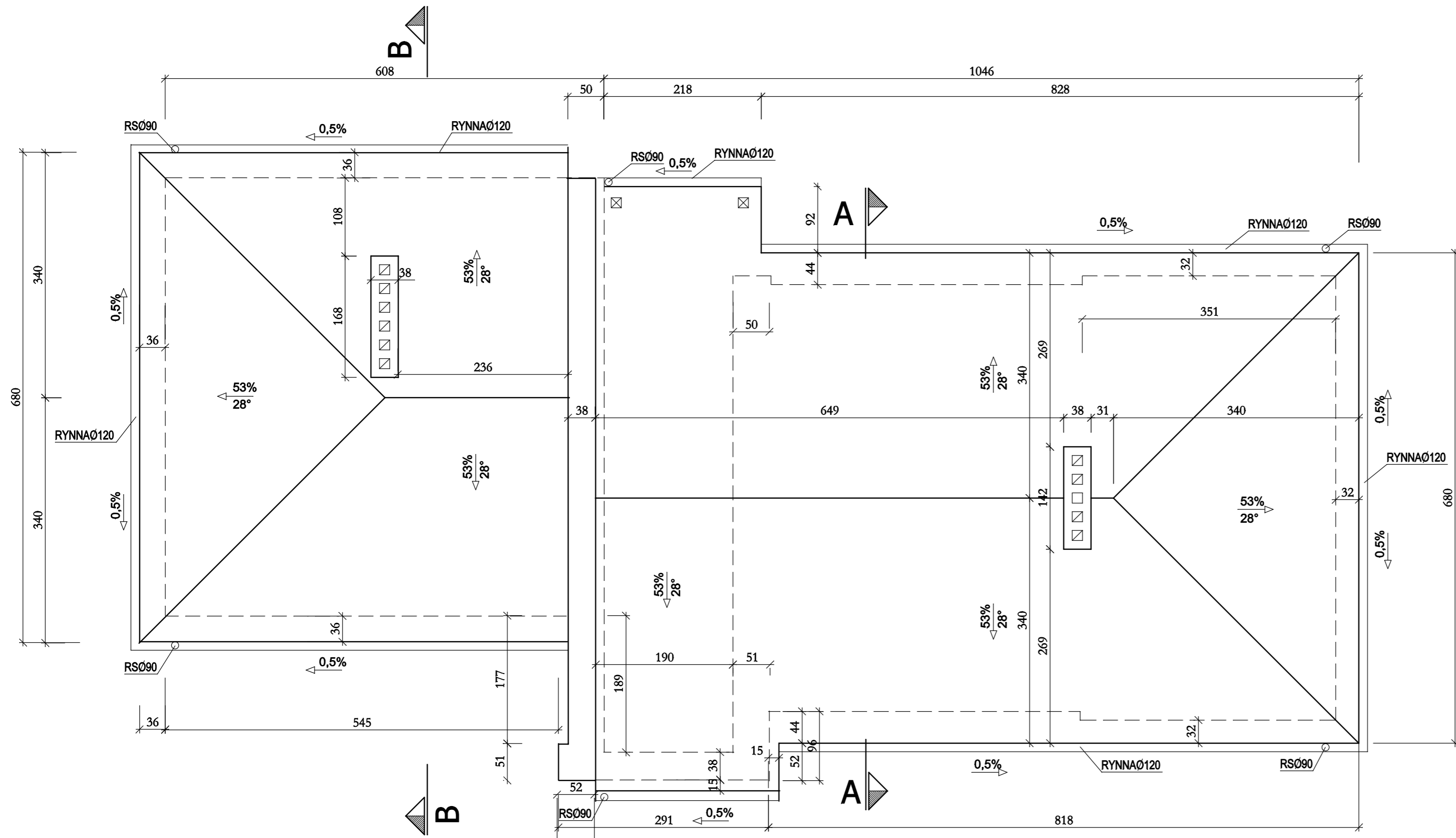
RZUT DACHU SKALA 1:50
