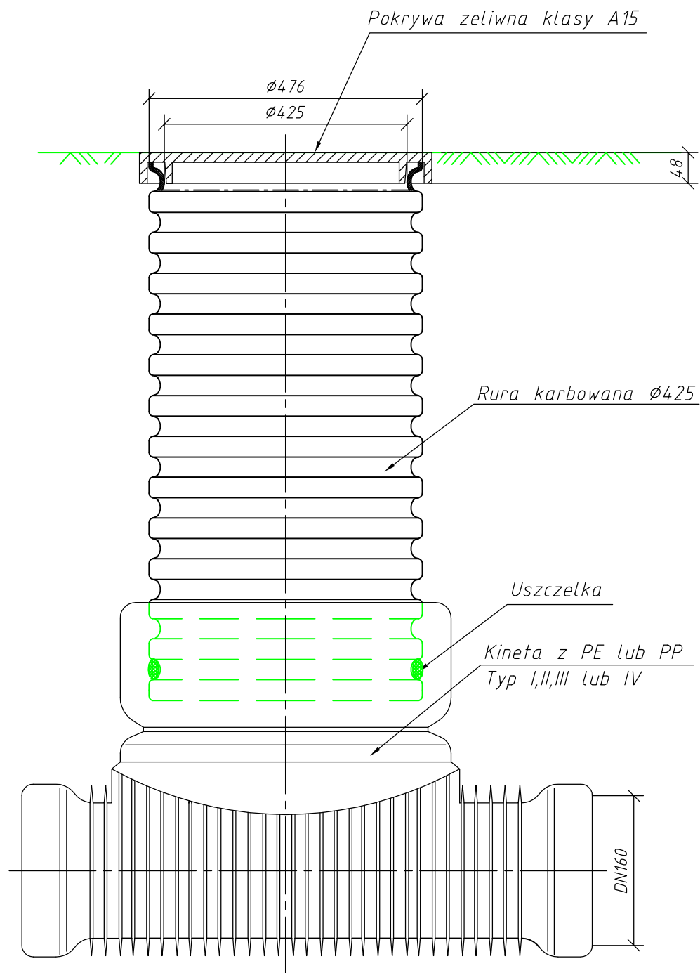
Studzienka inspekcyjna \varnothing 425 z pokrywa zeliwna klasy A15
