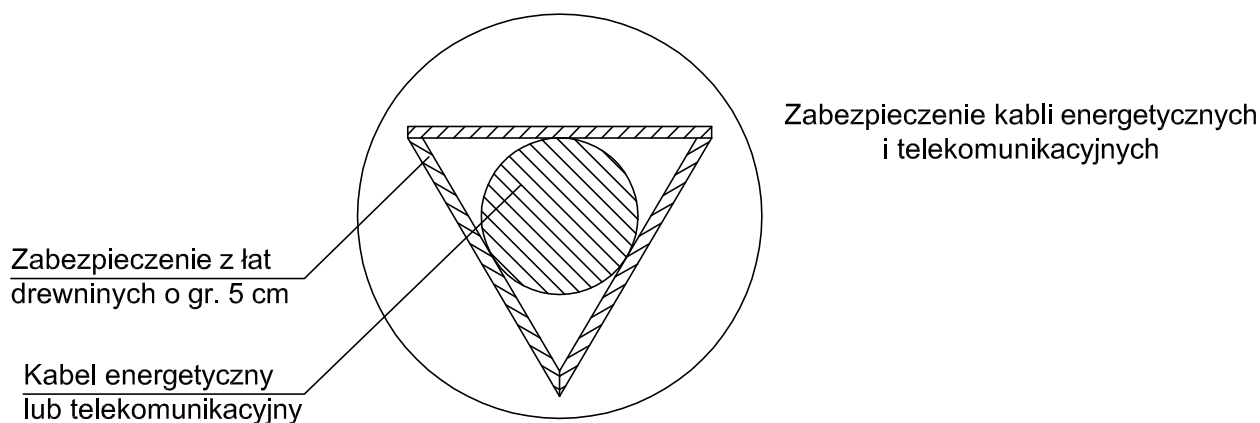
Przekrój A-A
